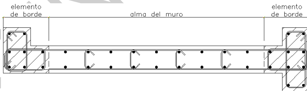
Fig. 21.1b Ejemplo de elementos de borde en muros
