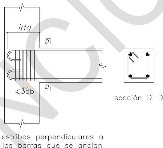
Fig. 12.5.3.c Caso con gancho estándar a 180^\circ en el que se puede multiplicar ldg por 0,8
