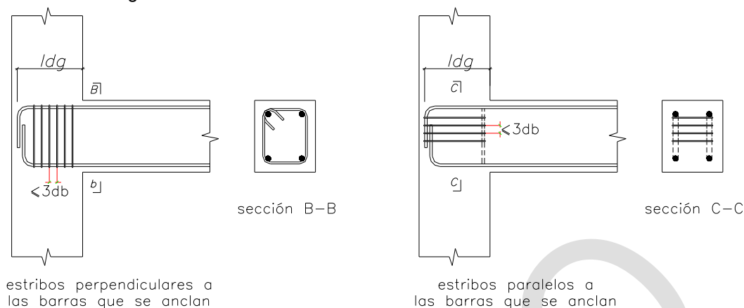
Fig. 12.5.3.b Casos con gancho estándar a 90^\circ en los que se puede multiplicar ldg por 0,8
